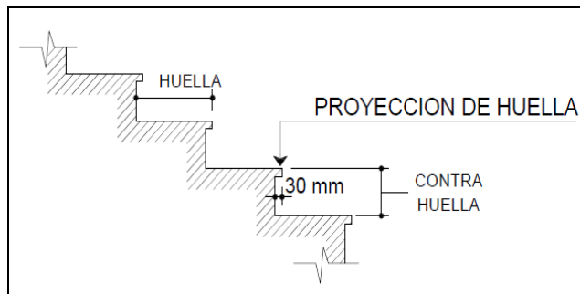
FIGURA 16 LARGO DE LA PROYECCIÓN DEL ESCALÓN
