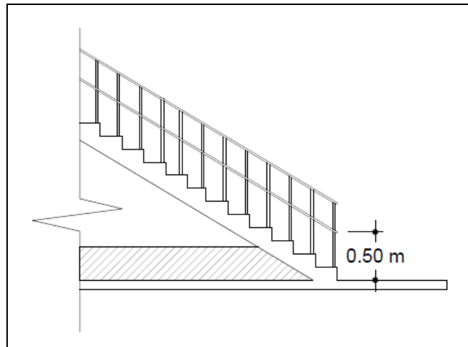
FIGURA 8 DOBLE PASAMANOS EN BARANDILLAS
