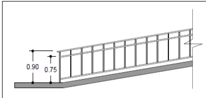
FIGURA 7 ALTURA DE PASAMANOS
