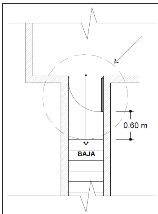
FIGURA 4 DETALLES TIPO DE PUERTAS DE ACCESO AL MEDIO DE CIRCULACIÓN VERTICAL
