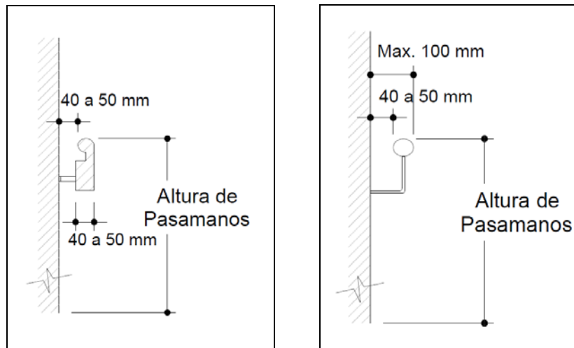
FIGURA 9 ESPACIO LIBRE ENTRE PASAMANOS Y PARED
