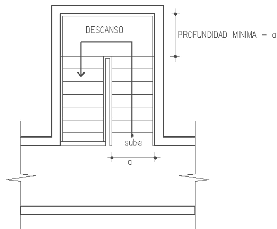
FIGURA 10 PROFUNDIDAD DE LOS DESCANSOS
