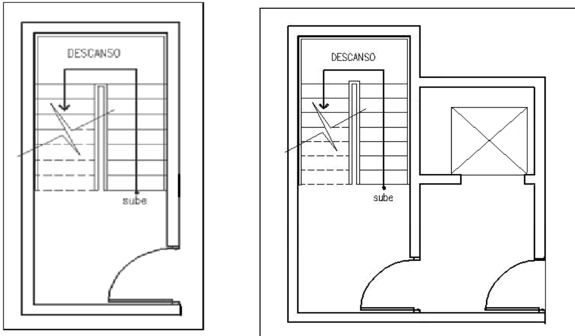
FIGURA 5 ÁREA DE ACCESO PROTEGIDA EN CIRCULACIÓN VERTICAL
