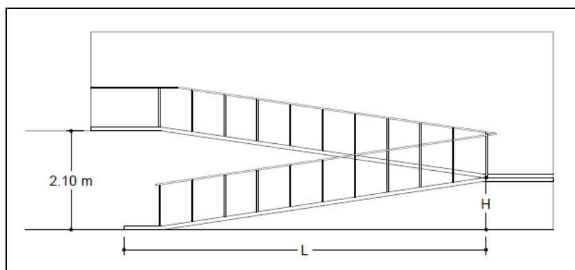
FIGURA 24 ALTURA LIBRE DE PISO A TECHO
