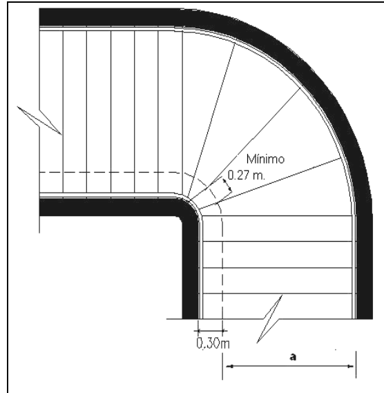
FIGURA 14 DETALLE ESCALERA MIXTA COMPENSADA
