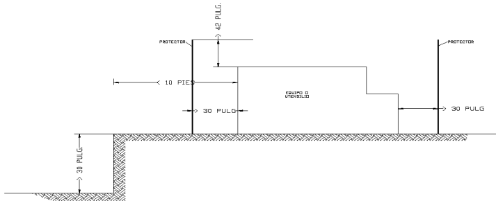
Figura C1 Instalación de Protector
